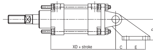
Type AFME Rear 90° Hinge
